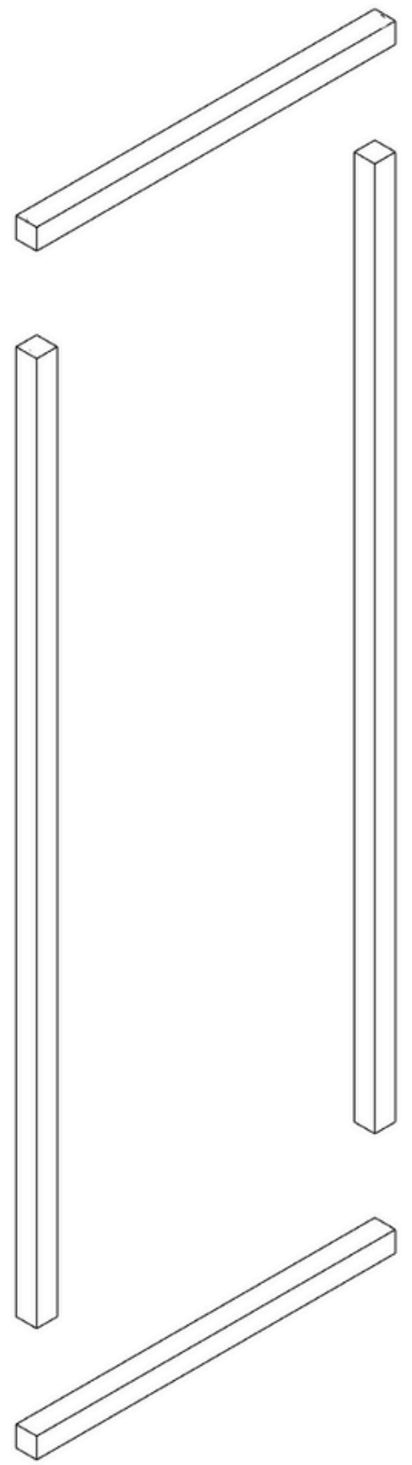
Stelkozijn kepers set (1x)
